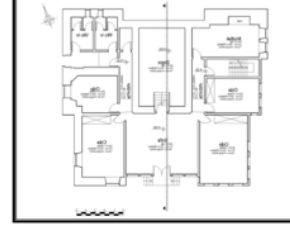
Çizim 7 Zemin kat planı
