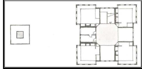
Çizim 4. Orta sofalı Plan tipi Safranbolu Gökçüoğlu evi (Sözen, 2001)
