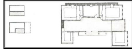
Çizim 2. Dış sofalı Plan tipi Kula Beyoğlu evi (Sözen, 2001)
