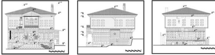
Karşloğlu konağı güney-doğu-batı cephe görünüşü
