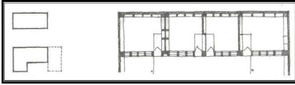
Çizim 1. Sofasız Plan tipi Antakya Kavuçuk evi (Sözen, 2001)
