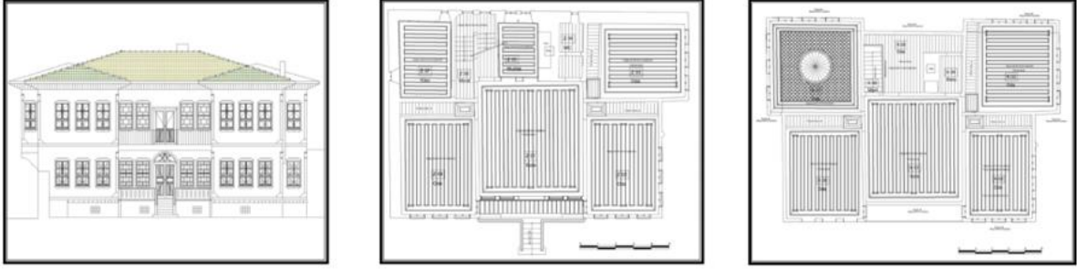
Çizim 15 Hayri İnal Konağı Restorasyon Projesi Teknik Çizimleri (Kaynak: Yozgat valiliği il özel idaresi)
