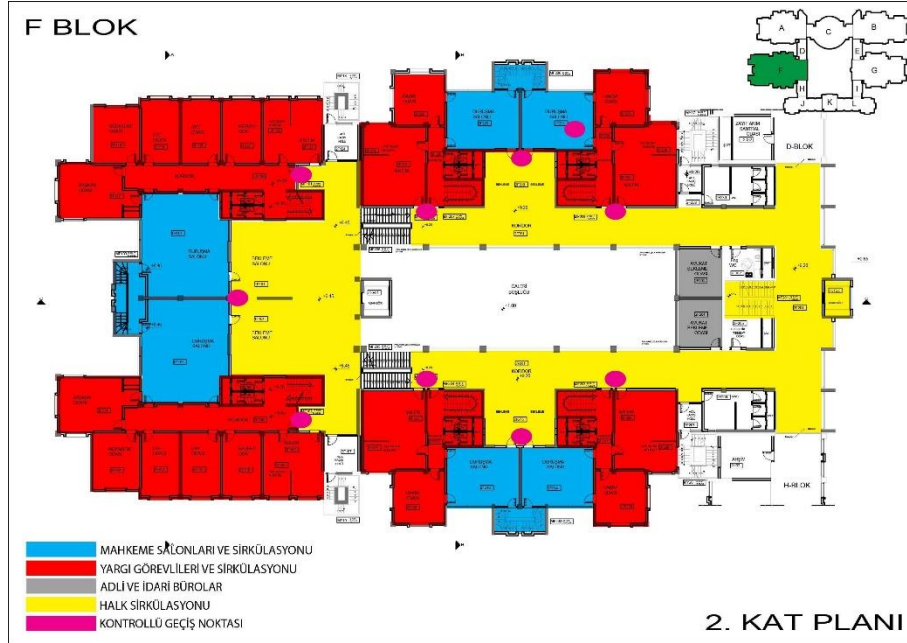
Şekil 7 - F Blok zemin ve normal kat ön plan - arka plan analizi
