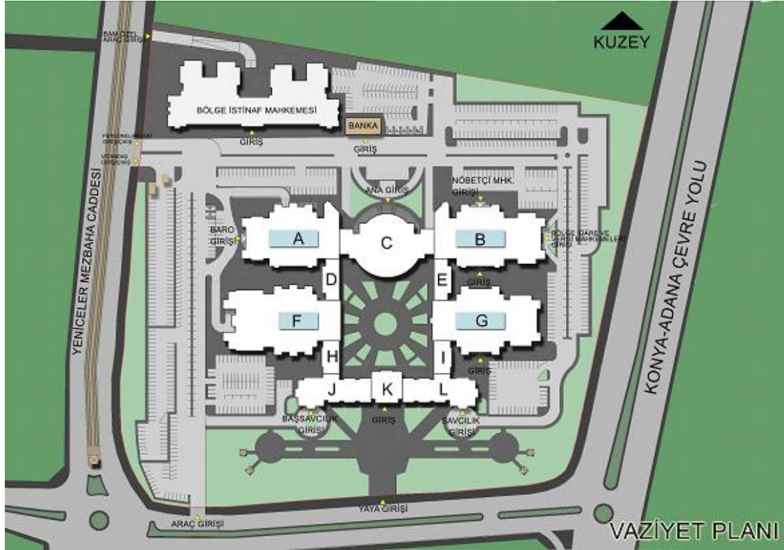
Şekil 5 – Konya Adliyesi vaziyet planı
