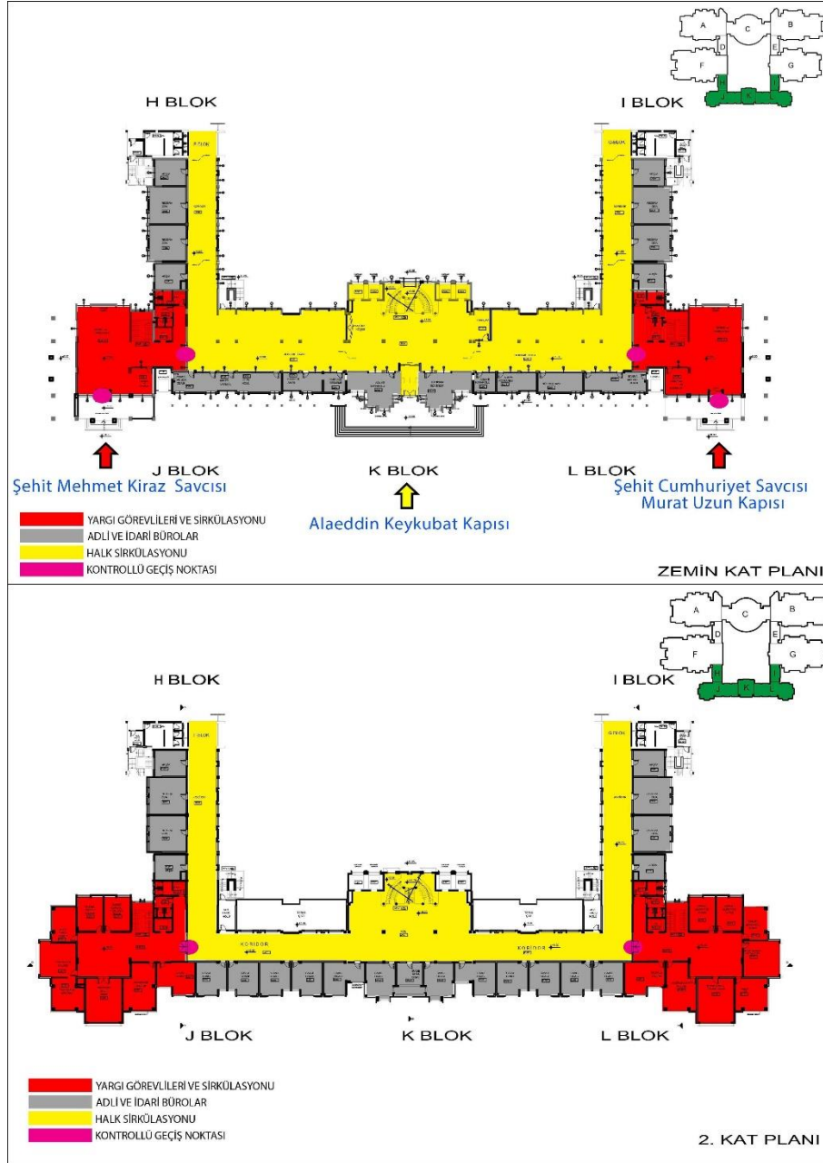
Şekil 11 - H-I-J-K-L bloklar zemin ve normal kat ön plan - arka plan analizi
