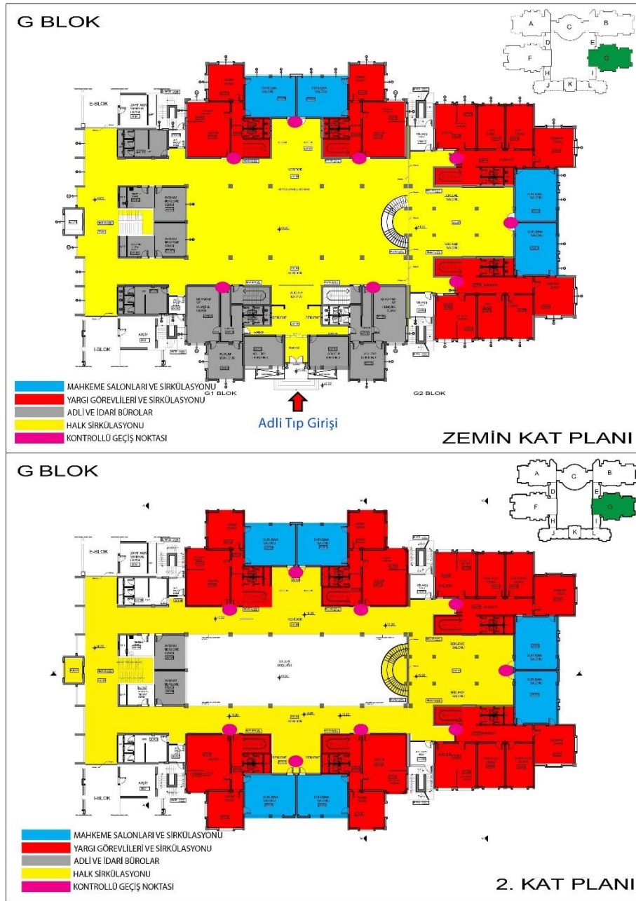
Şekil 9 - G Blok zemin ve normal kat ön plan - arka plan analizi
