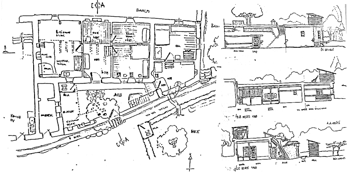
Şekil 11. Muammer Kutlutan Evi planı, cephe ve kesitleri (Kutlutan, 1997: 87-88)
