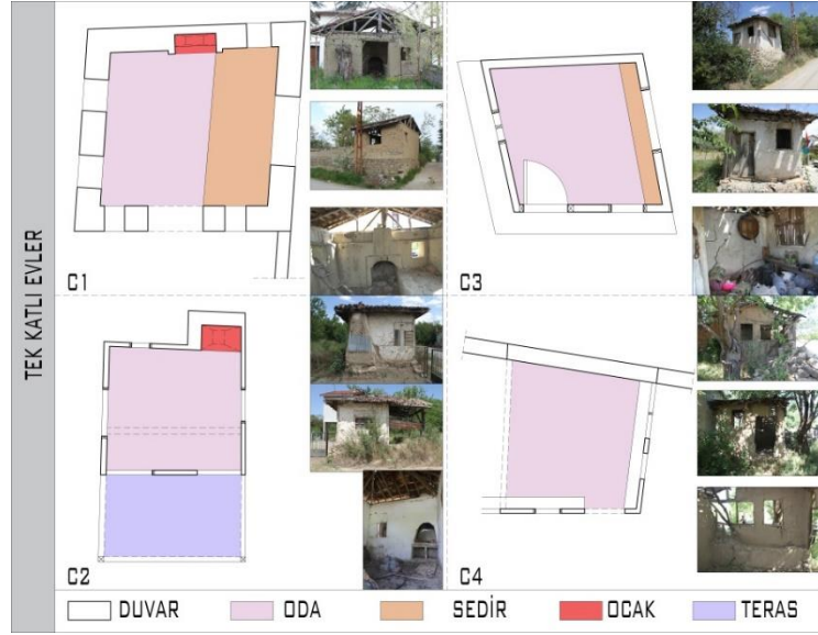
Şekil 22. Tek katlı bağ evleri plan tipi
