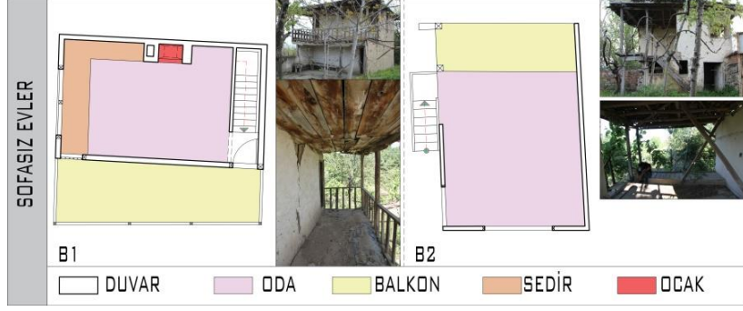
Şekil 21. Bağ evleri sofasız plan tipi
