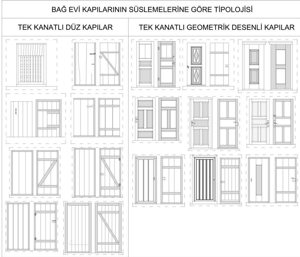
Şekil 14. Tokat bağ evlerinde ahşap kapılar
