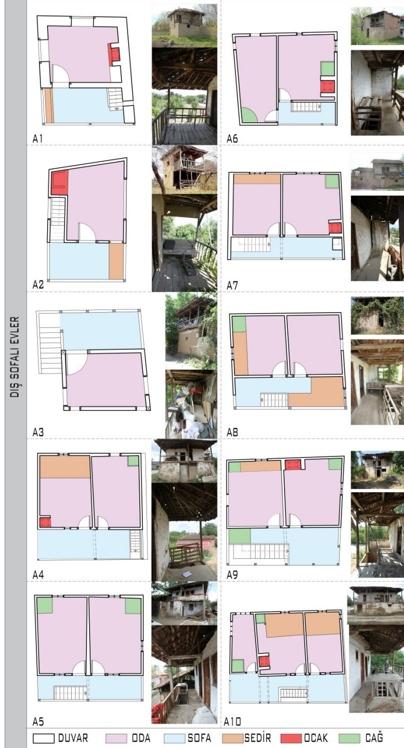
Şekil 20. Bağ evleri dış sofalı plan tipi
