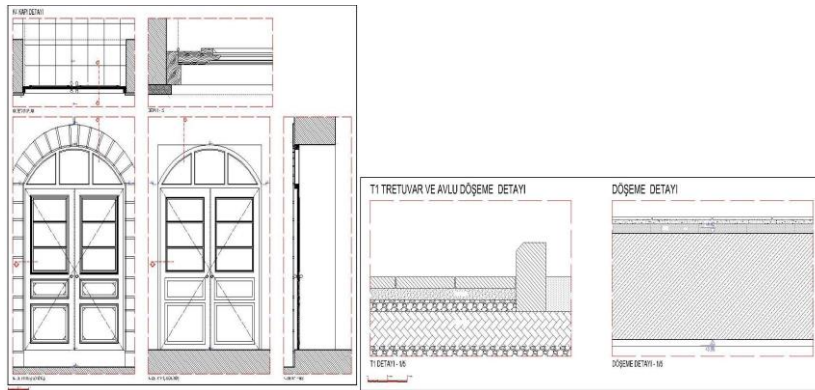
Çizim-31,32: Muş Eski Hükümet Konağı Giriş Kapısı ve Zemin Detayları (Ş. Öztürk)
