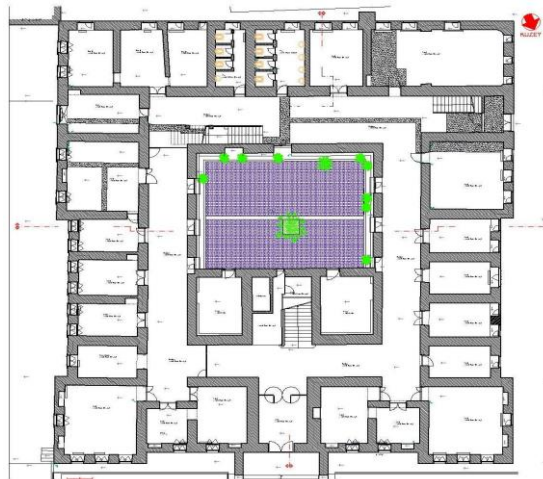
Çizim-05: Muş Eski Hükümet Konağı Rölöve Zemin Kat Planı (Ş. Öztürk)
