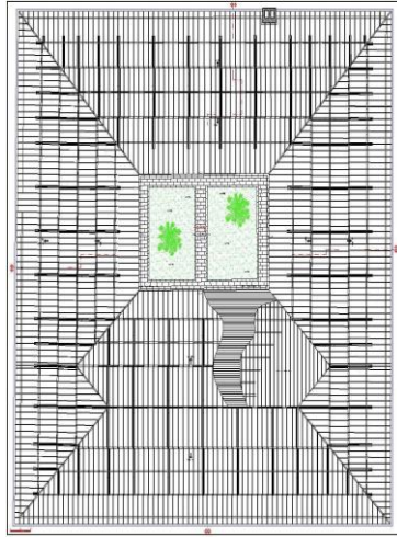
Çizim-17: Muş Eski Hükümet Konağı Restorasyon Çatı Planı (Ş. Öztürk) Fotoğraf-44: Muş Eski Hükümet Konağı Onarım Öncesi Çatı Görünüşü (Ş. Öztürk)
