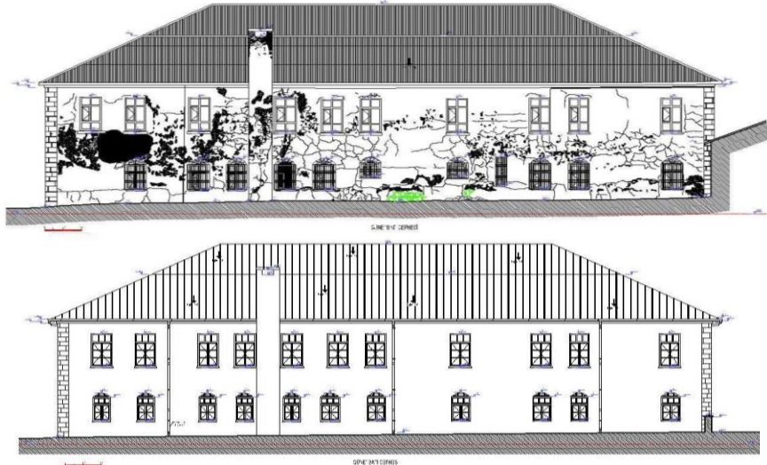
Çizim-12,13: Muş Eski Hükümet Konağı Güney Cephe Rölöve-Restorasyonu (Ş. Öztürk)
