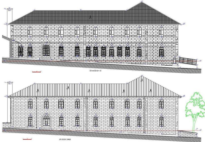
Çizim-15,16: Muş Eski Hükümet Konağı Doğu Cephe Rölöve-Restorasyonu (Ş. Öztürk)
