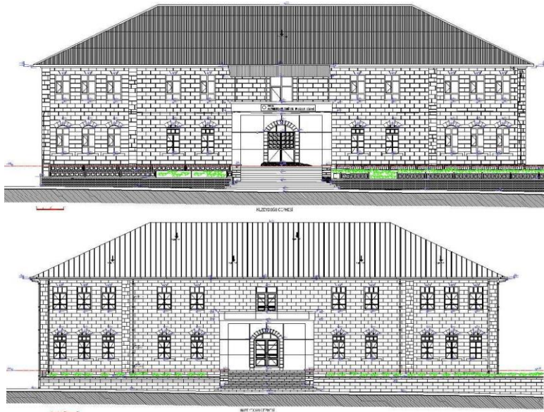
Çizim-10,11: Muş Eski Hükümet Konağı Kuzey Cephe Rölöve-Restorasyonu (Ş. Öztürk)
