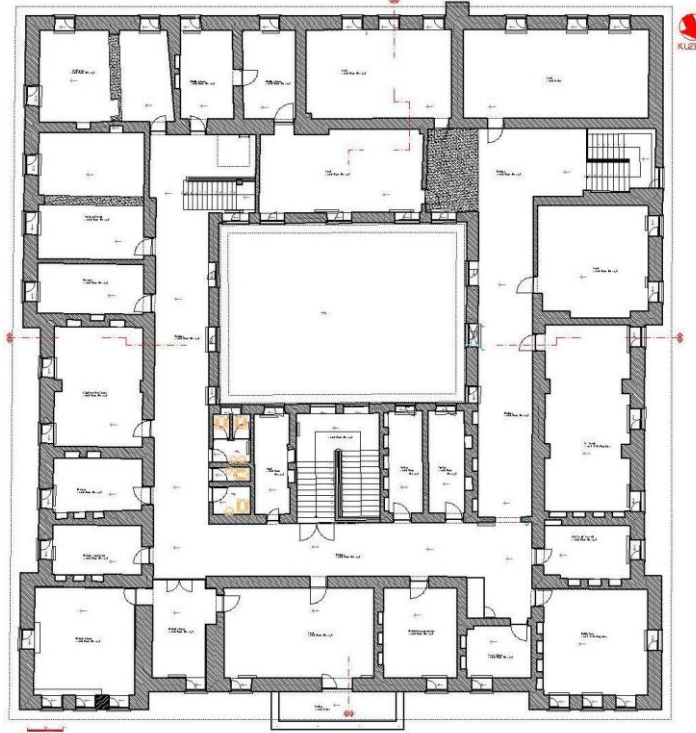
Çizim-07: Muş Eski Hükümet Konağı Rölöve Üst Kat Planı (Ş. Öztürk)
