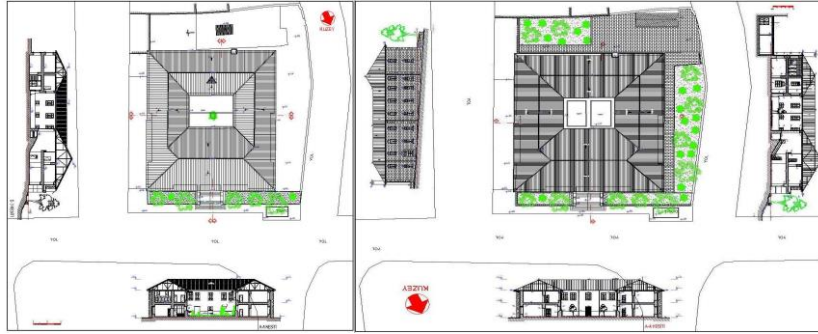
Çizim-01,02: Muş Eski Hükümet Binası Rölöve ve Restorasyon Vaziyet Planı (Ş. Öztürk)
