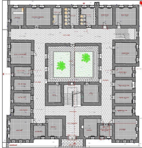
Çizim-06: Muş Eski Hükümet Konağı Restorasyon Zemin Kat Planı (Ş. Öztürk)
