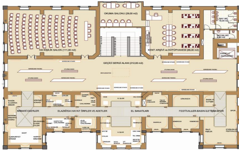
Çizim-29: Eski Hükümet Konağı Kent Müzesi Üst Kat Planı (Ş. Öztürk)
