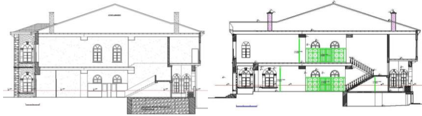
Çizim-19,20: Eski Elazığ Hükümet Konağı Rölöve-Restorasyon A-A En Kesitleri (Ş. Öztürk)
