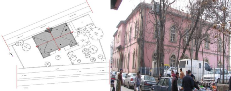
Çizim-1:Eski Elazığ Hükümet Konağı Vaziyet Rölöve Planı (Ş. Öztürk)
