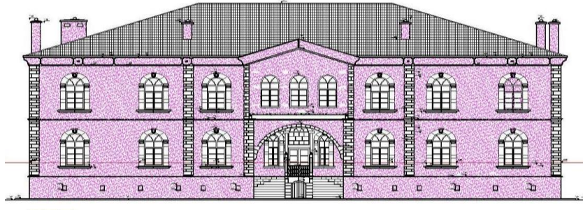
Çizim-15,16: Eski Elazığ Hükümet Konağı Güney Cephe Rölöve- Restorasyonu (Ş. Öztürk)
