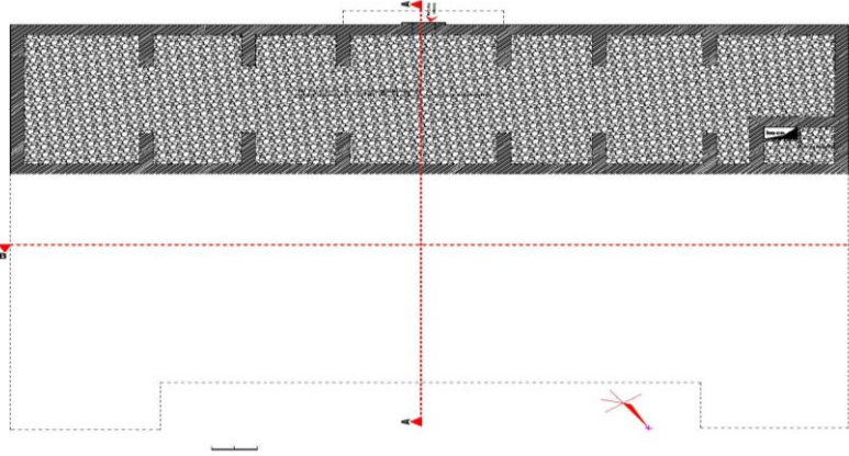
Çizim-2: Eski Elazığ Hükümet Konağı Bodrum Kat Rölöve Planı (Ş. Öztürk)
