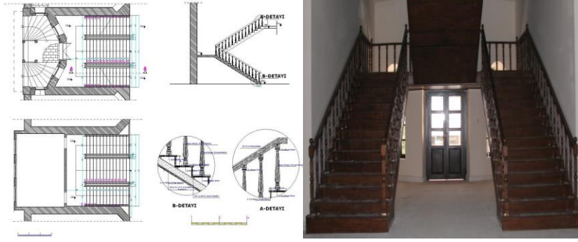
Çizim-5:Merdiven Plan ve Detayları; Fotoğraf-20: Eski Hükümet Konağı Merdiven Onarım Sonrası Görünüşü (Ş. Öztürk)
