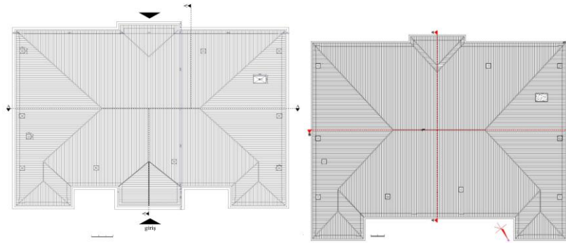
Çizim-17,18: Eski Elazığ Hükümet Konağı Güney Cephe Rölöve-Restorasyonu (Ş. Öztürk)
