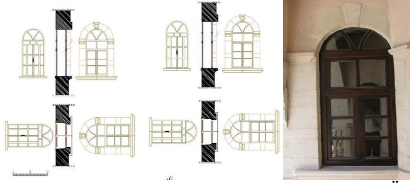
Çizim-23,24: Eski Hükümet Konağı Zemin ve Üst Kat Pencere Detayları (Ş. Öztürk)
