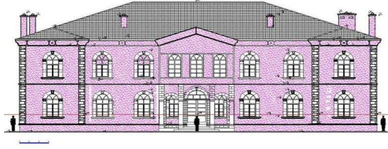
Çizim-8,9: Eski Elazığ Hükümet Konağı Kuzey Cephe Rölöve-Restorasyonu (Ş. Öztürk)
