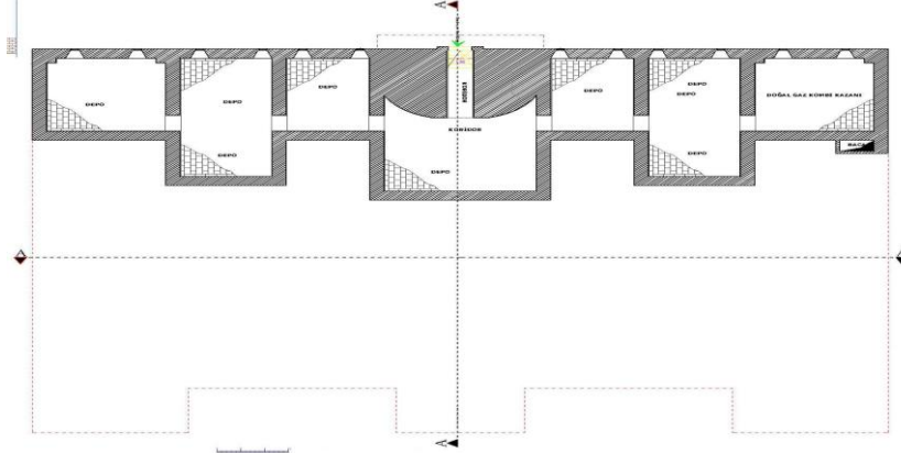
Çizim-3: Eski Elazığ Hükümet Konağı Bodrum Kat Rölöve Planı (Ş. Öztürk)
