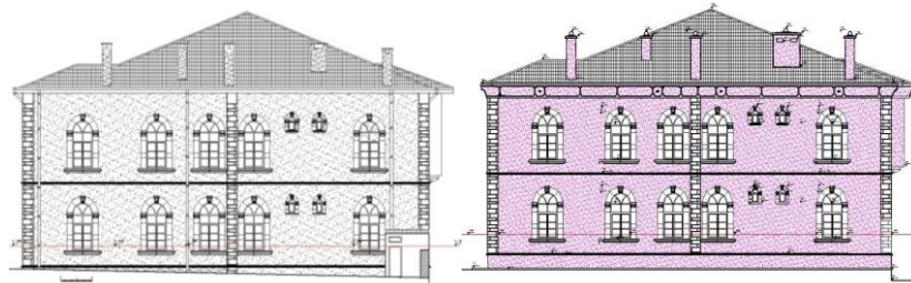
Çizim-12,13: Eski Elazığ Hükümet Konağı Batı Cephe Rölöve-Restorasyonu (Ş. Öztürk)
