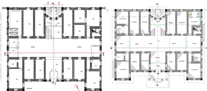
Çizim-3,4: Eski Elazığ Hükümet Konağı Zemin Kat Rölöve-Restorasyon Planları (Ş. Öztürk)
