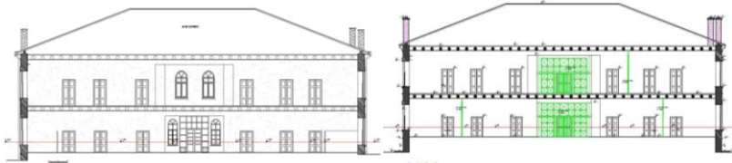
Çizim-21,22: Eski Elazığ Hükümet Konağı Rölöve-Restorasyon B-B Boy Kesitleri (Ş. Öztürk)
