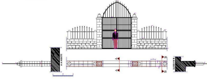
Çizim-25: Eski Hükümet Konağı Giriş Kapısı Detayları (Ş. Öztürk)
