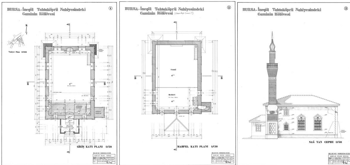
Şekil 4. Tahtaköprü Hamidiye Camisinin 1982 Tarihli Rölövesi (Tahtaköprü Belediyesi Arşivi)
