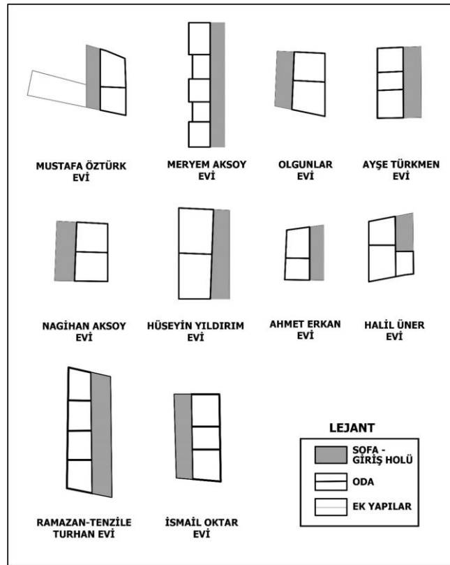
Şekil 9. Tahtaköprü'deki Dış Sofalı Evlerin Plan Şemaları
