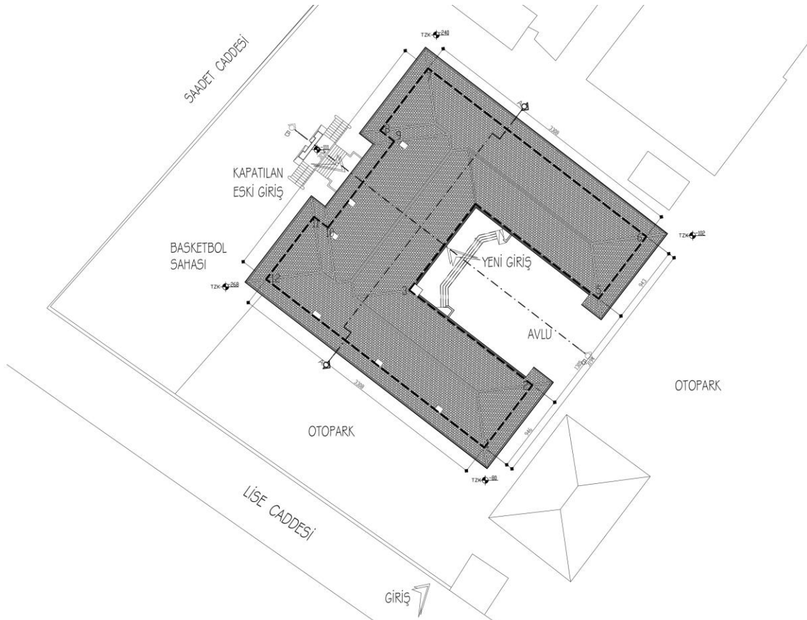
Resim 3. Samsun Olgunlaşma Enstitüsü Vaziyet Planı (Mustafa Güner Ofisi)
