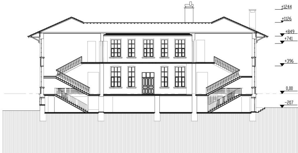
Resim 15. Samsun Olgunlaşma Enstitüsü A-A Kesiti (Mustafa Güner Ofisi)
